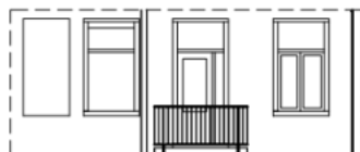
Voorgevel woning
