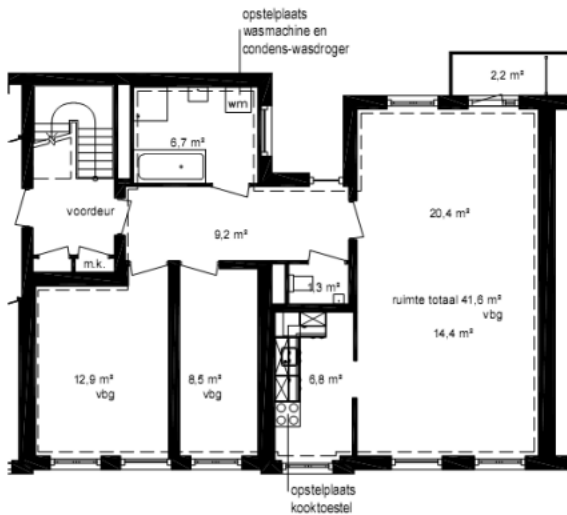
Plattegrond woning
