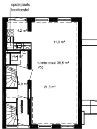
Plattegrond woning
