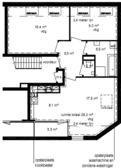
Plattegrond woning
