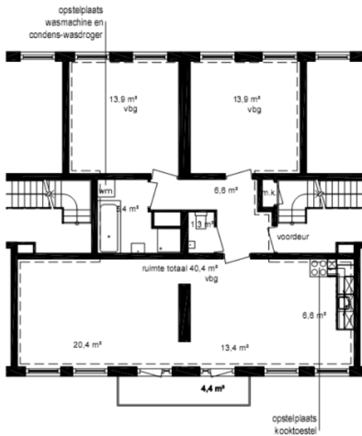
Plattegrond woning
