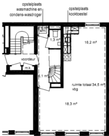
Plattegrond woning
