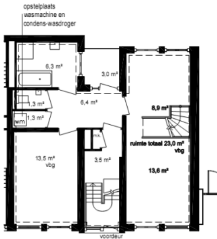
Plattegrond woning
