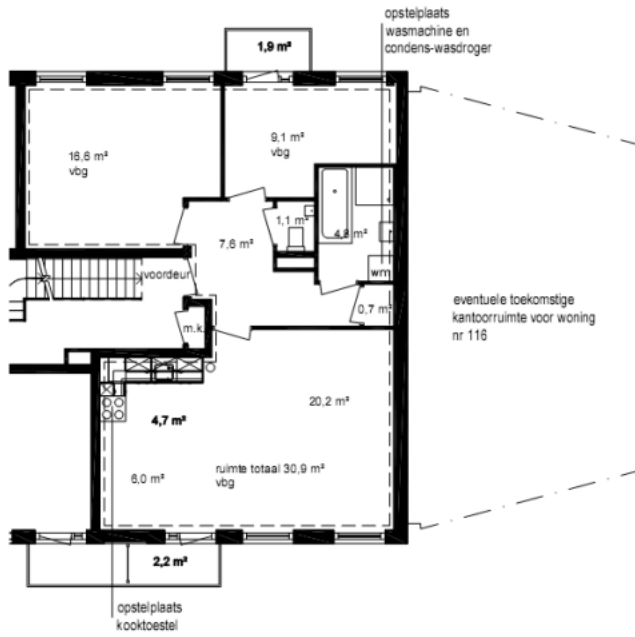
Plattegrond woning
