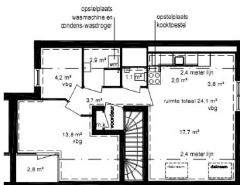
Plattegrond woning
