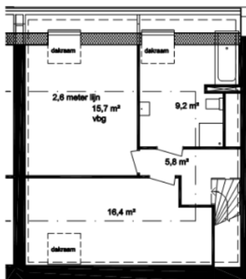
Plattegrond woning
