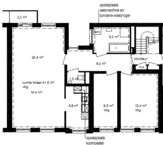
Plattegrond woning
