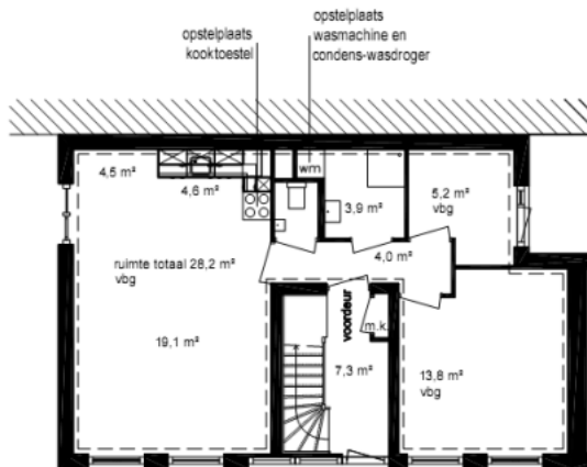
Plattegrond woning
