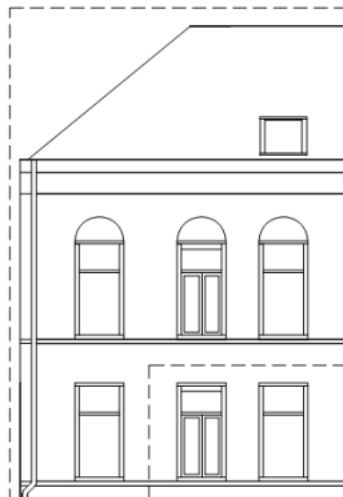
Voorgevel woning
