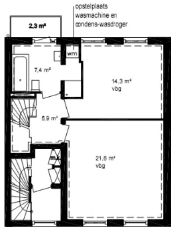
Plattegrond bovenverdieping
