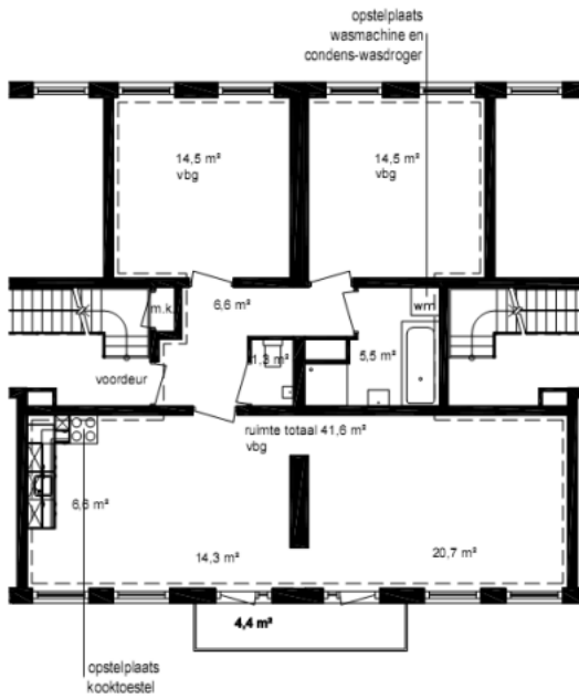
Plattegrond woning
