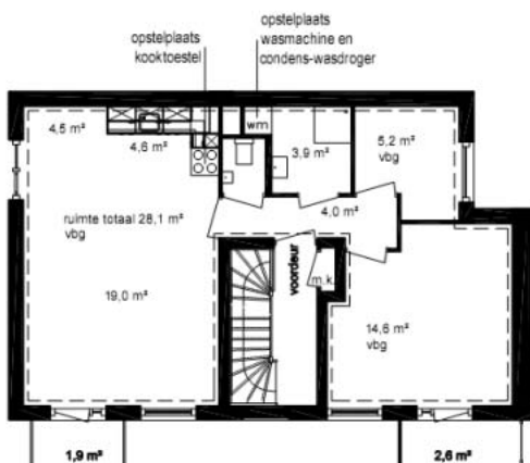
Plattegrond woning
