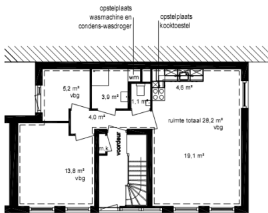
Plattegrond woning
