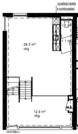
Plattegrond bedrijfsruimte
