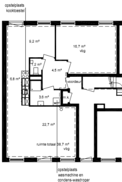
Plattegrond woning
