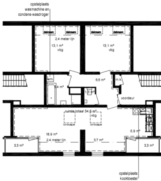
Plattegrond woning
