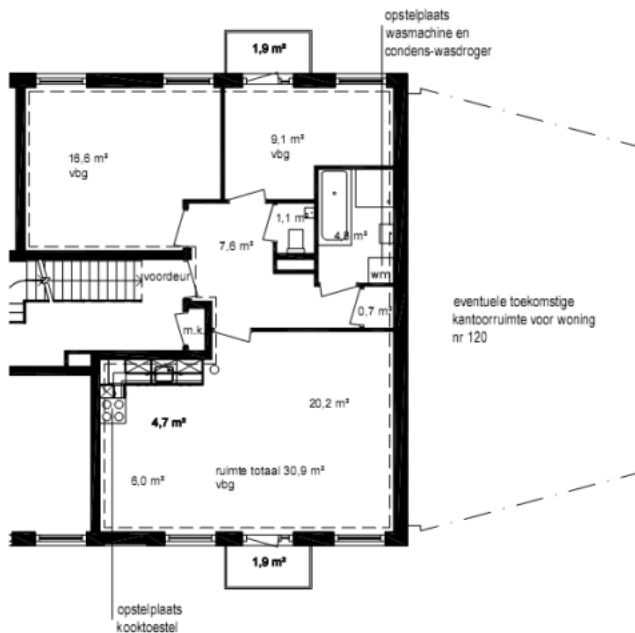
Plattegrond woning
