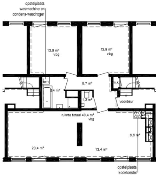
Plattegrond woning
