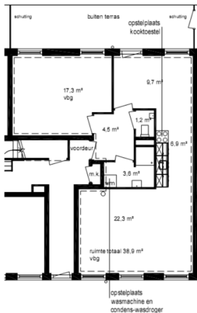
Plattegrond woning
