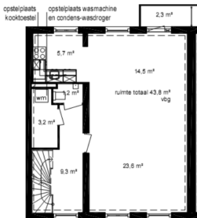
Plattegrond woning
