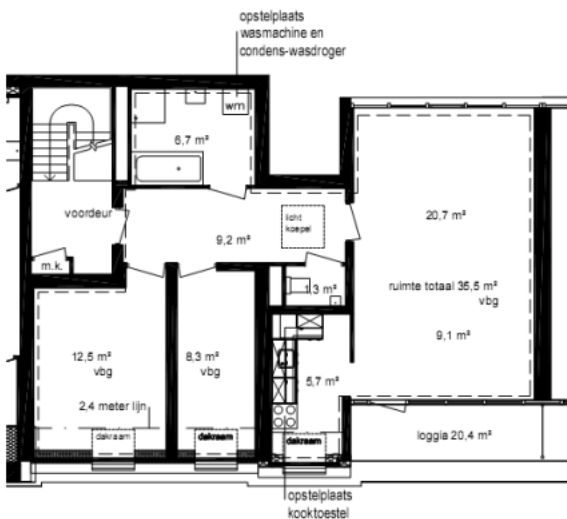
Plattegrond woning
