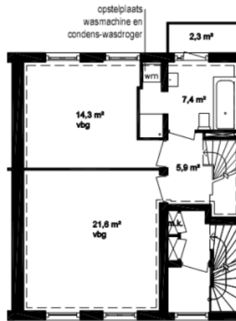
Plattegrond bovenverdieping
