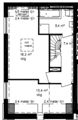
Plattegrond bovenverdieping
