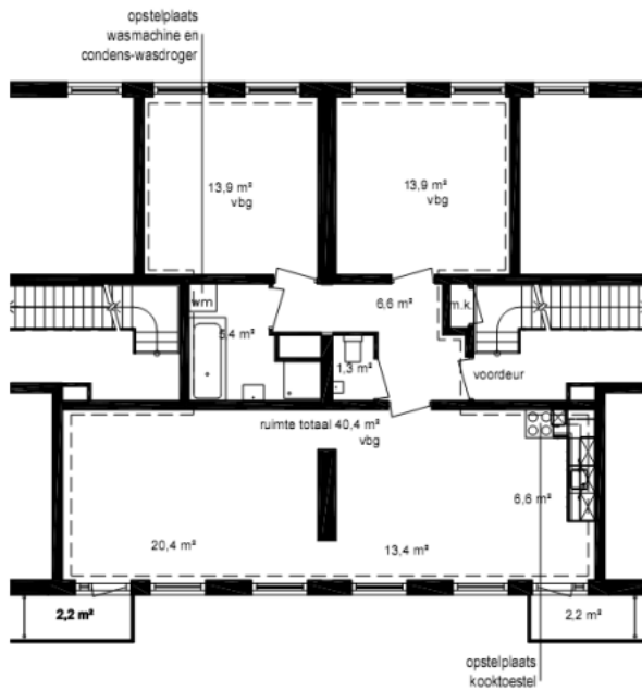
Plattegrond woning
