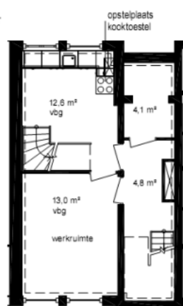
Plattegrond onderverdieping
