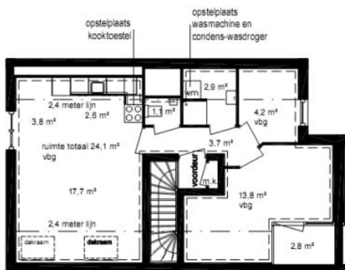
Plattegrond woning
