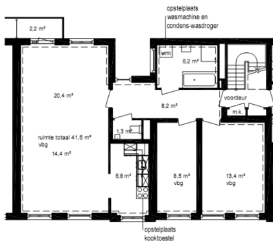
Plattegrond woning
