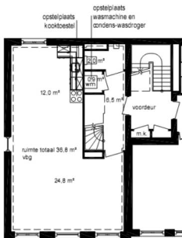
Plattegrond woning
