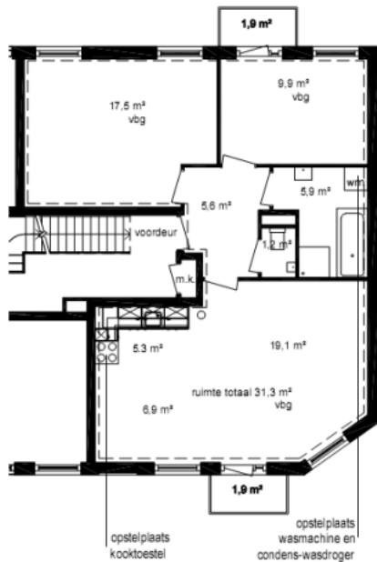
Plattegrond woning
