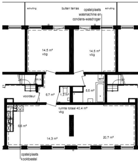
Plattegrond woning
