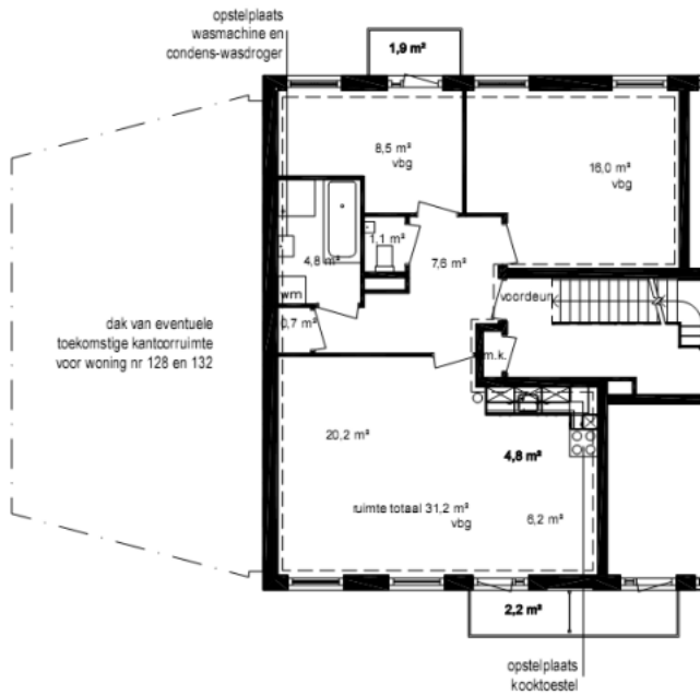
Plattegrond woning
